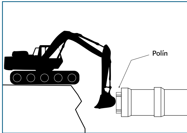
Figura 5.17 Palanca mecánica y polín
