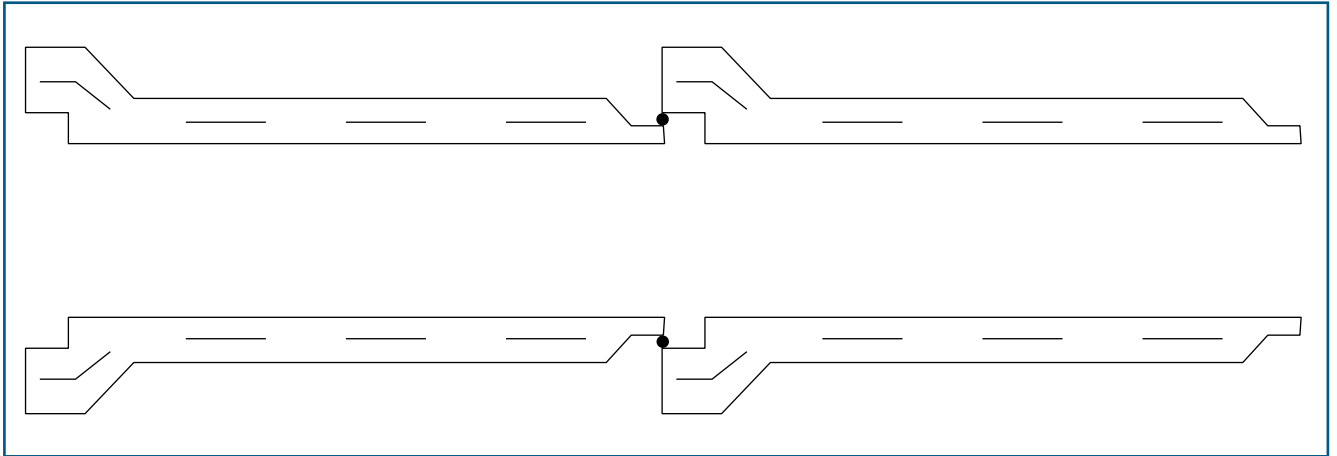
Figura 5.25 Posición correcta el roce parejo de la junta de hule en toda la periferia de la campana
