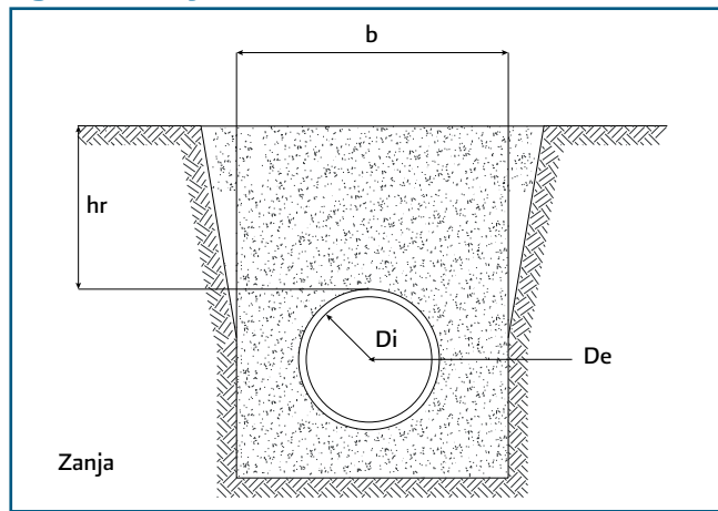
Figura 5.4 Zanja
