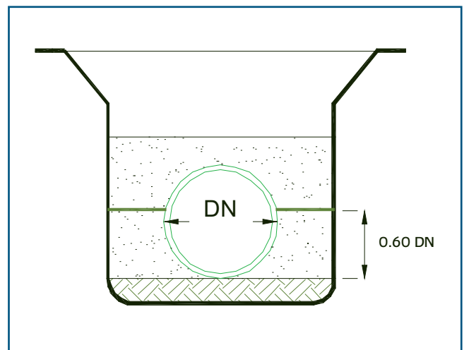
Figura 3.16 Instalación tipo 2
