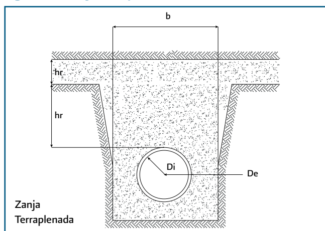
Figura 5.5 Zanja terraplenada
