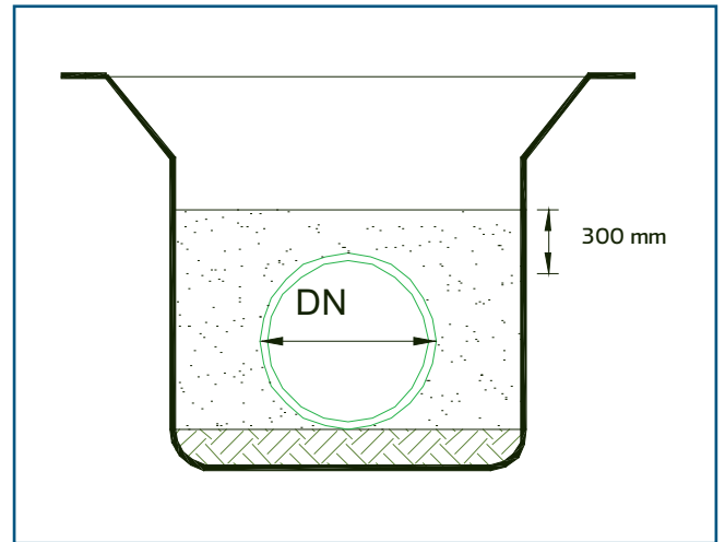
Figura 3.15 Instalación tipo 1
